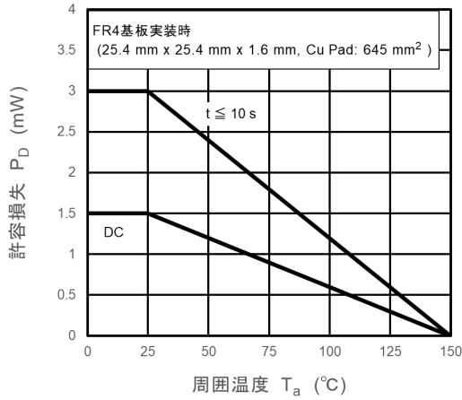
図 8.13 P_D - T_a
