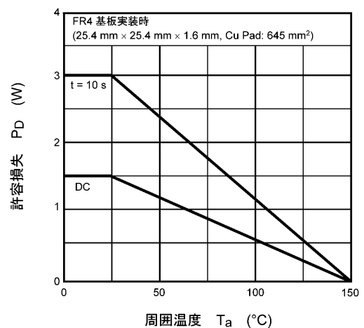
図 7.12 P_D - T_a
