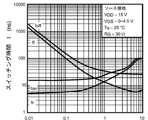
図 7.10 t - I_D
