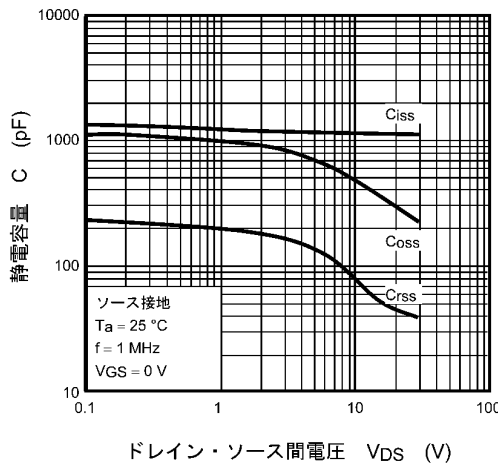
図 8.9 C - V_{DS}
