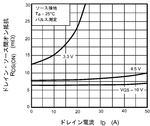
図 7.5 R_{DS(ON)} - I_D
