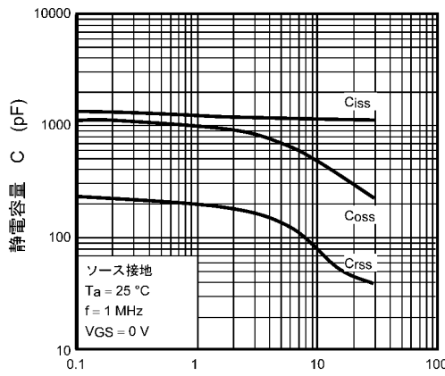
図 7.9 C - V_{DS}
