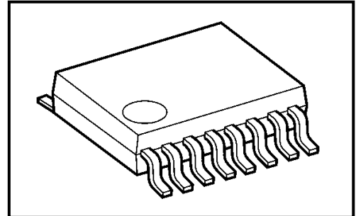
P-TSSOP16-0505-0.65-001 質量 : 0.06 g (typ.)
