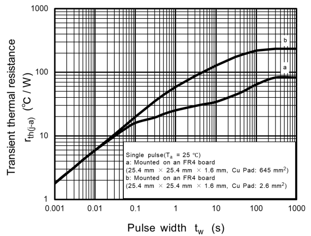
Fig. 9.12 r_{th(j-a)} - t_w
