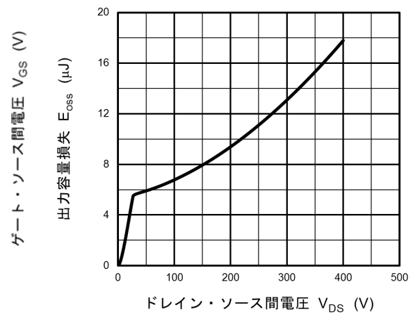
図 8.12 E_{oss} - V_{DS}
