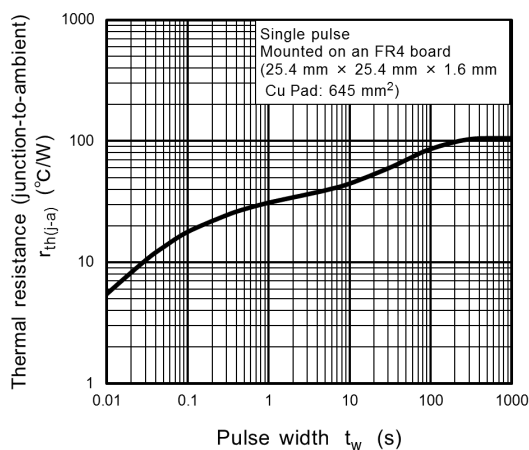
Fig. 9.4 r_{th} - t_w
