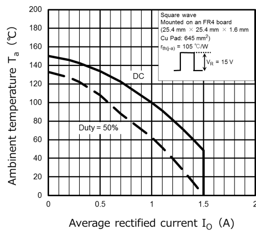
Fig. 9.6 T_a - I_O
