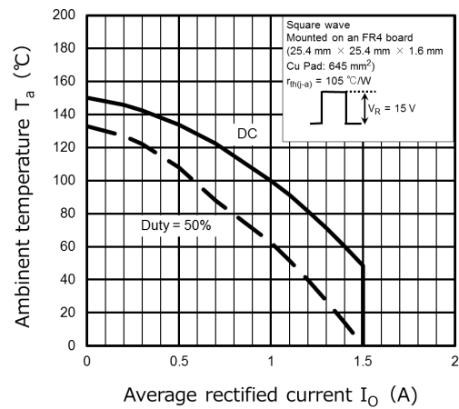
図 9.6 T_a - I_O
