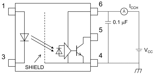
Fig. 12.1.3 I_{CCH} Test Circuit
