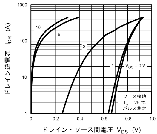
図 8.10 I DR - V DS
