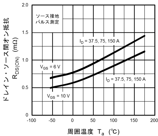
図 8.9 R DS(ON) - T a
