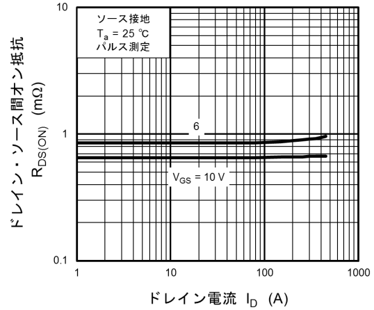
図 8.8 R DS(ON) - I D
