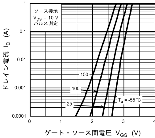
図 8.7 I D - V GS
