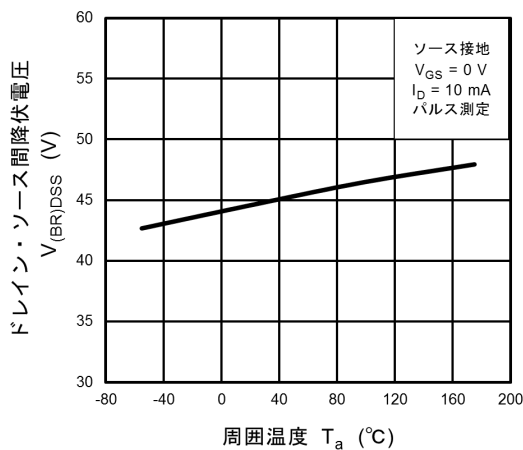
図 8.11 V (BR)DSS - T a
