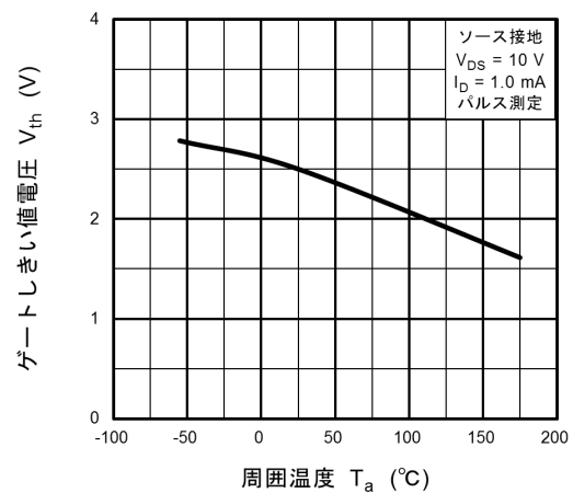
図 8.12 V th - T a
