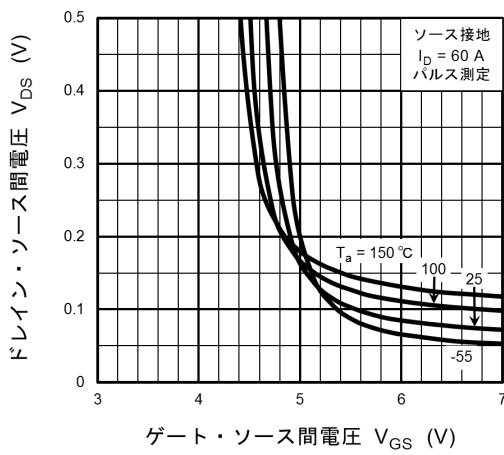
図 8.3 V_{DS} - V_{GS}
