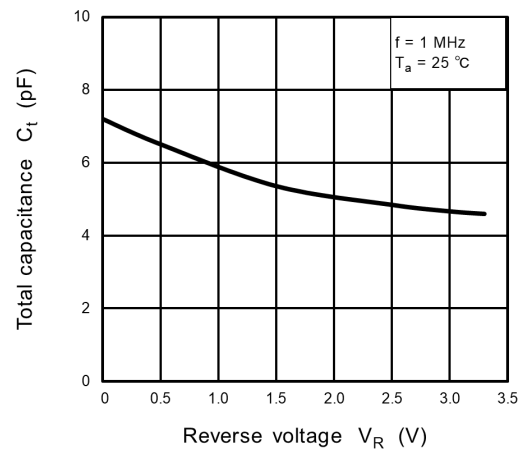
Fig. 9.2 C_t - V_R
