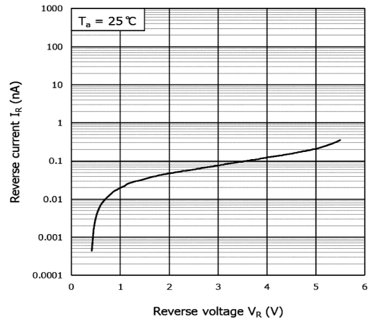
Fig. 9.2 I_R - V_R
