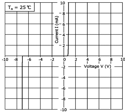
Fig. 9.1 I - V
