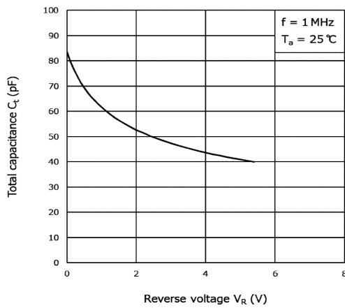
Fig. 9.3 C_t - V_R
