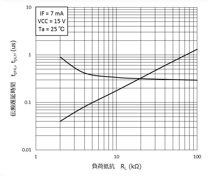
t_{pLH} , t_{pHL} - R_L
