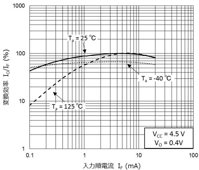
I_O/I_F - I_F
