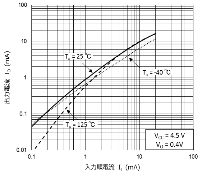
I_O - I_F
