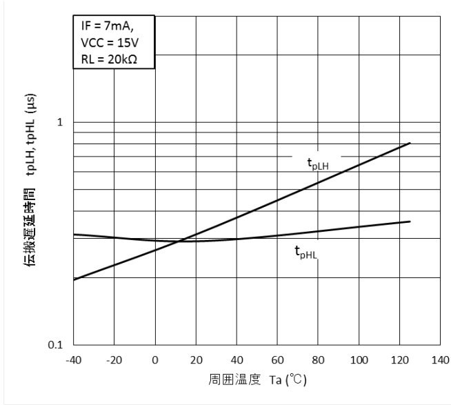
t_{pLH} , t_{pHL} - T_a
