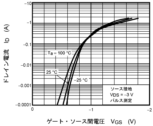
図 8.2 I_D - V_{GS}
