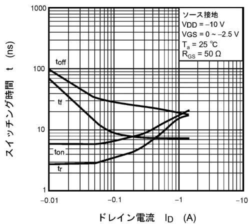
図 8.11 t - I_D
