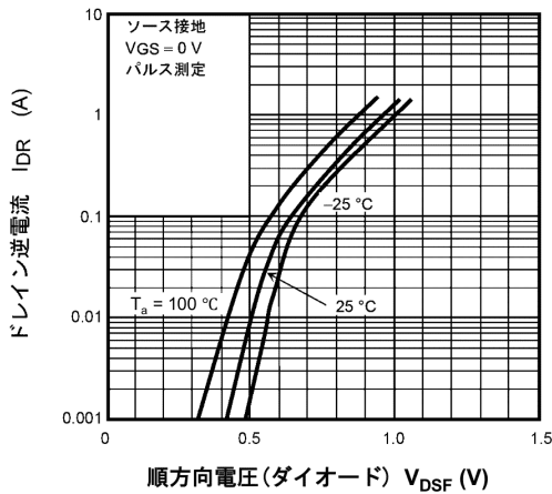
図 8.9 I_{DR} - V_{DSF}
