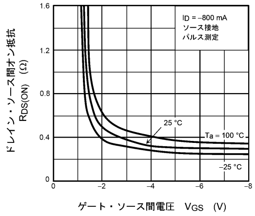
図 8.4 R_{DS(ON)} - V_{GS}
