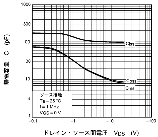
図 8.10 C - V_{DS}
