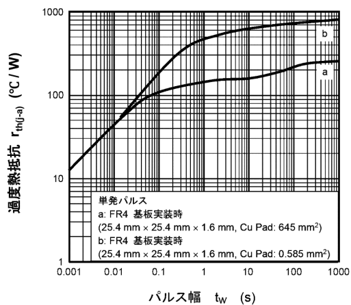
図 8.13 r_{th(j-a)} - t_w
