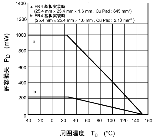
図 9.13 P_D - T_a
