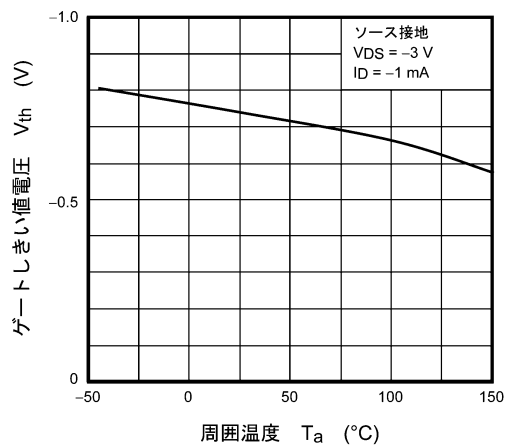
図 9.6 V_{th} - T_a
