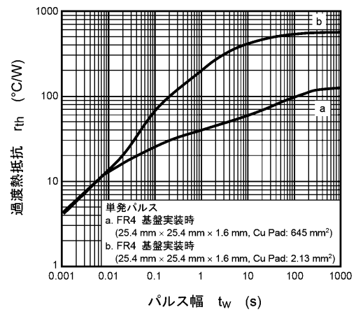
図 9.12 r_{th} - t_w
