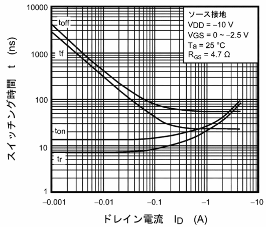
図 9.10 t - I_D
