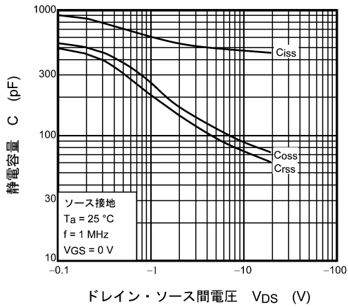
図 9.9 C - V_{DS}
