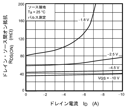
図 9.4 R_{DS(ON)} - I_D
