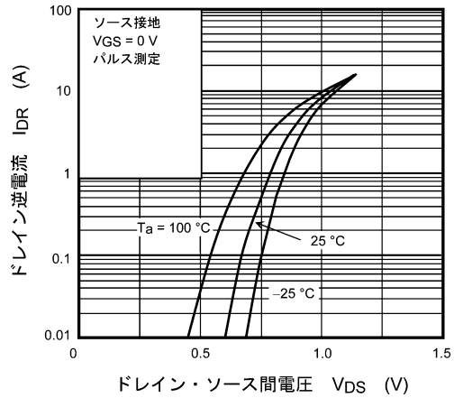
図 9.8 I_{DR} - V_{DS}
