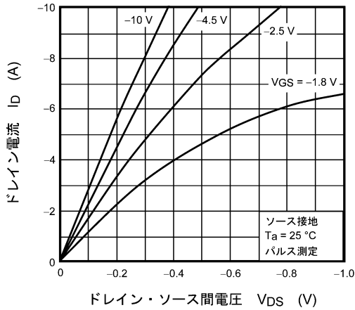
図 9.1 I_D - V_{DS}
