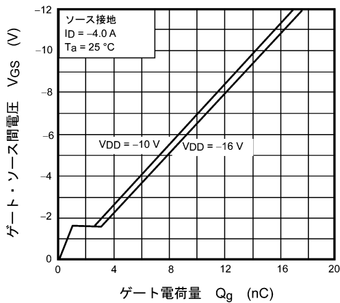
図 9.11 ダイナミック入力特性
