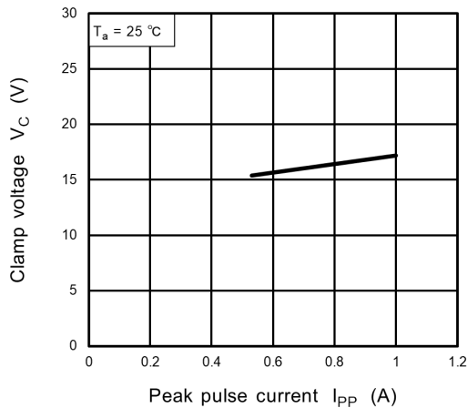
図 6.2.1 V_C - I_{PP}
