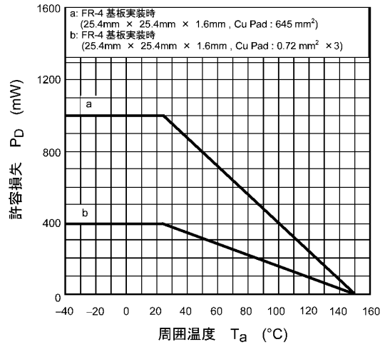
図 9.14 P_D - T_a
