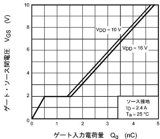
図 9.12 ダイナミック入力特性
