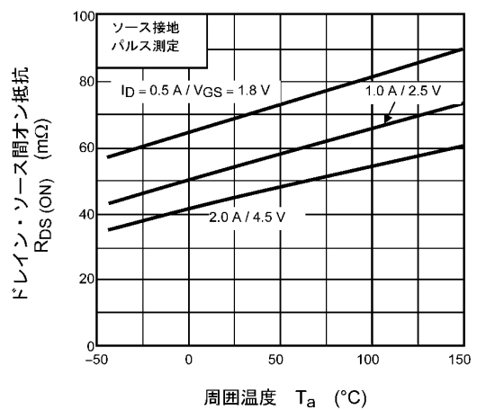
図 9.6 R_{DS(ON)} - T_a
