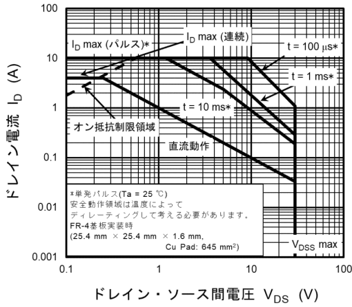
図 9.15 安全動作領域
