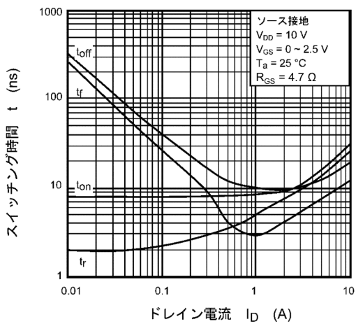
図 9.11 t - I_D
