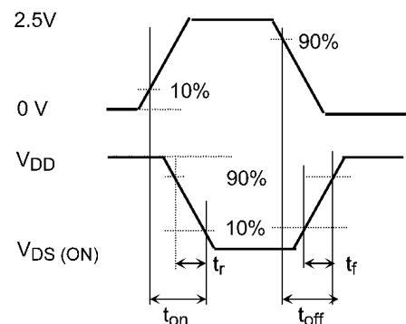
図 7.3.2 入力波形/出力波形
