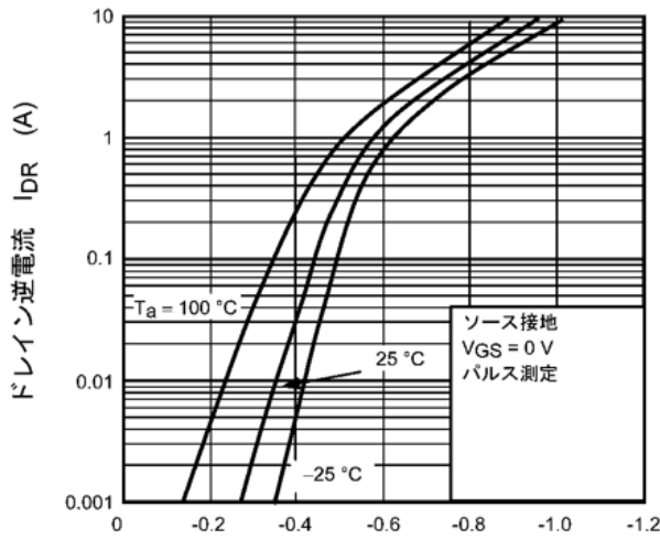
図 9.9 I_{DR} - V_{DS}
