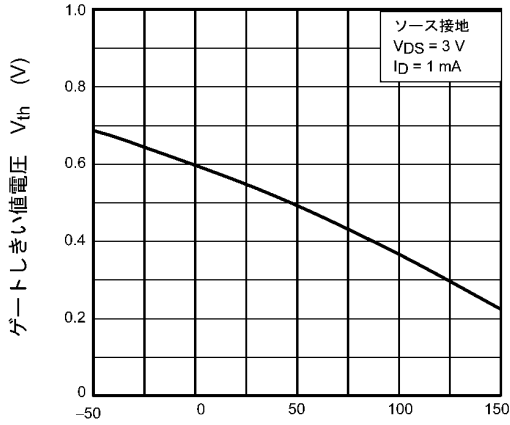
図 9.7 V_{th} - T_a
