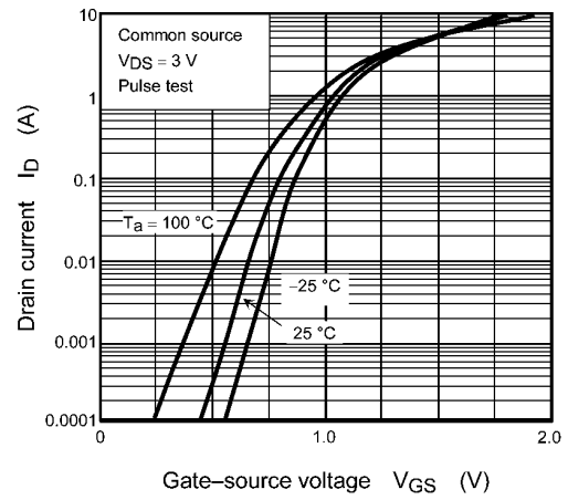
Fig. 9.2 I_D - V_{GS}
