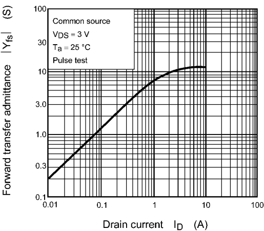
Fig. 9.8 |Y_{fs}| - I_D
