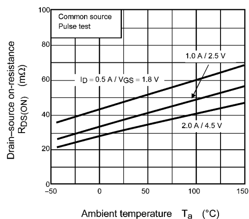
Fig. 9.6 R_{DS(ON)} - T_a
