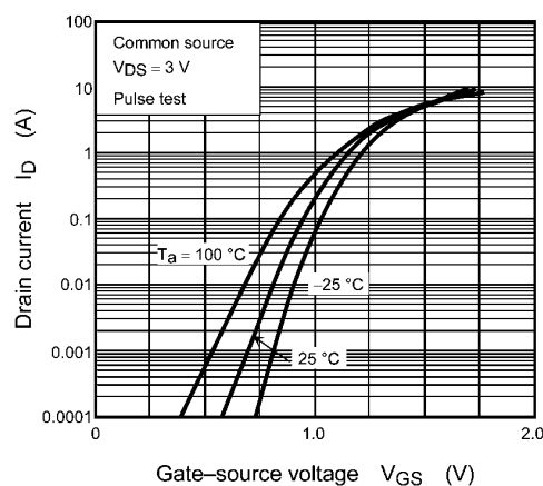
Fig. 9.2 I_D - V_{GS}
