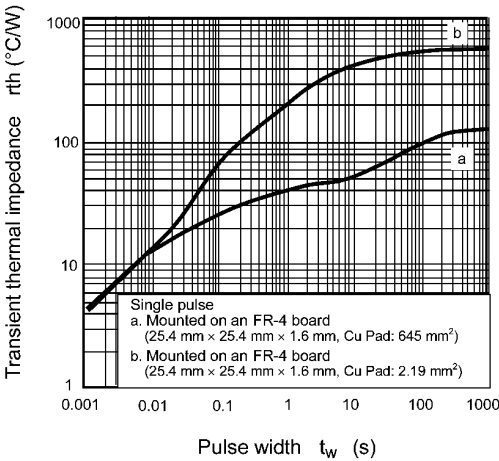
Fig. 9.13 r_{th} - t_w
