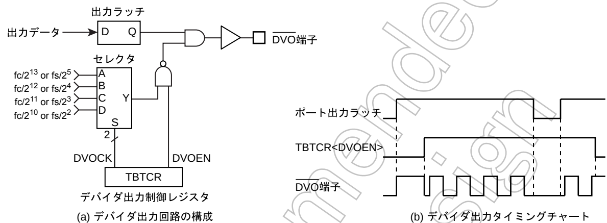
図 6-3 デバイダ出力
