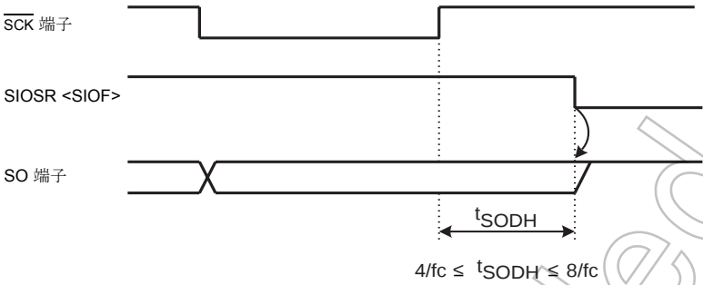
図 10-8 送信終了時のデータ保持時間
