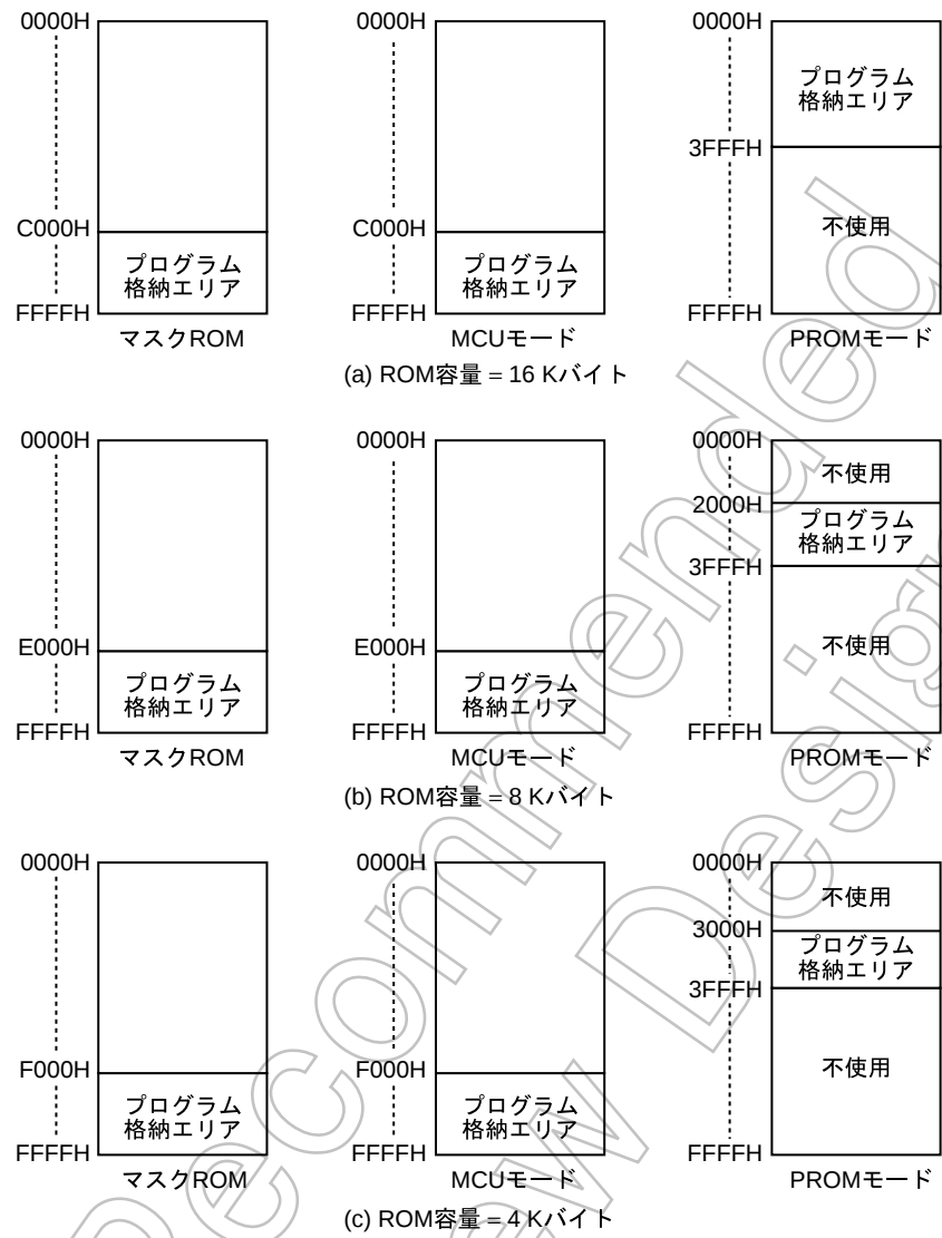
図 14-1 プログラム格納エリア
