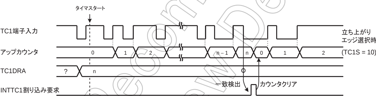
図 8-4 イベントカウンタモード タイミングチャート
