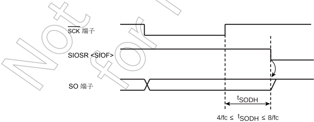
図 10-17 送受信終了時のデータ保持時間
