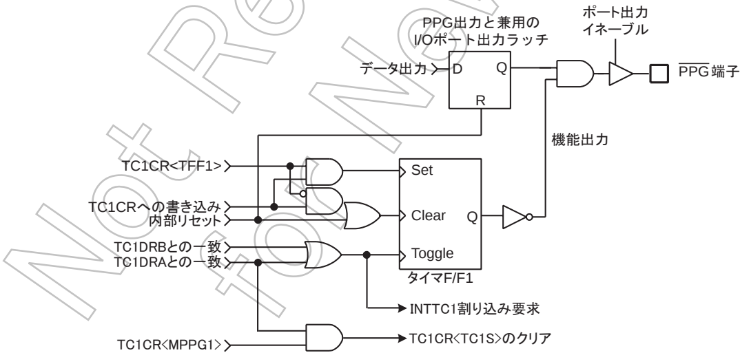
図 8-7 PPG 出力
