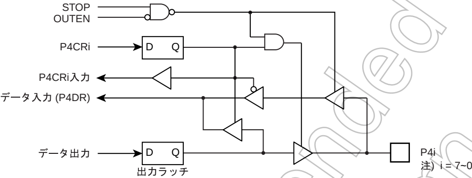
図 5-6 P4 ポート
