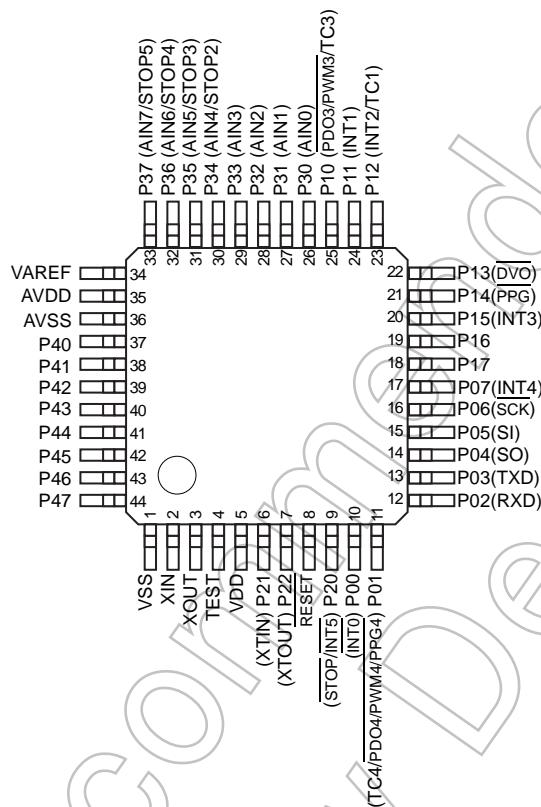
図 1-1 ピン配置図
