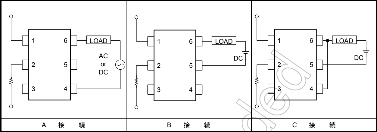
接続回路図
