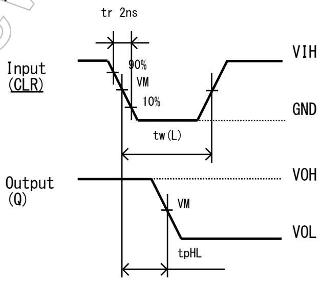
図 4 t_{pHL}, t_w(L)
