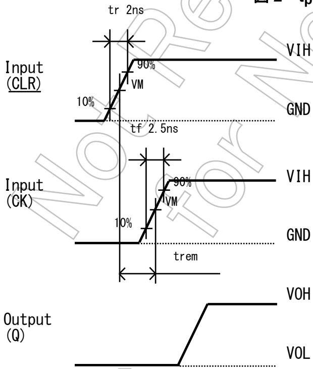
図 3 trem
