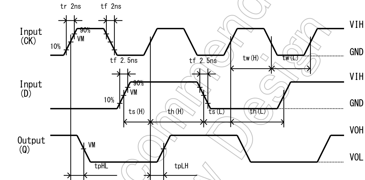
図 2 t_{pLH}, t_{pHL}
