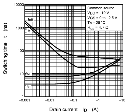
Fig. 9.10 t - I_D
