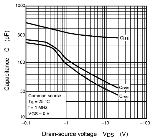
Fig. 9.9 C - V_{DS}
