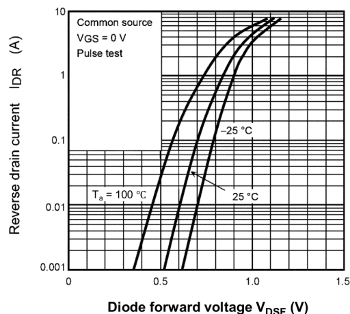
Fig. 9.8 I_{DR} - V_{DSF}
