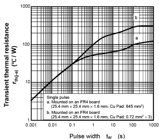
Fig. 9.12 r_{th(j-a)} - t_w
