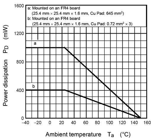
Fig. 9.13 P_D - T_a
