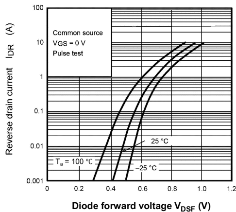
Fig. 9.9 I_{DR} - V_{DSF}
