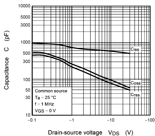
Fig. 9.10 C - V_{DS}
