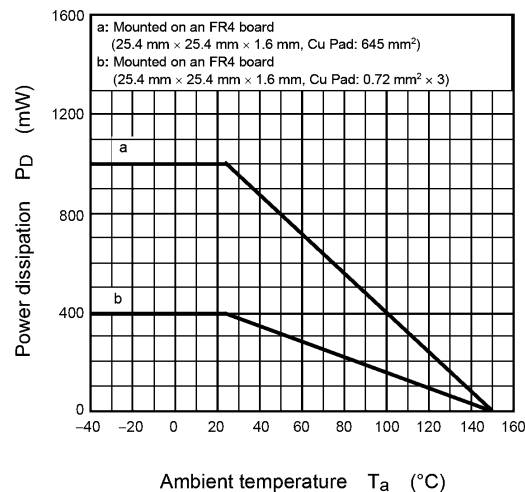
Fig. 9.14 P_D - T_a
