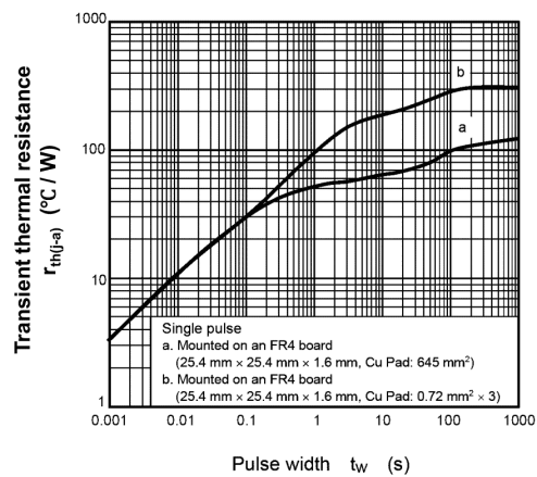
Fig. 9.13 r_{th(j-a)} - t_w
