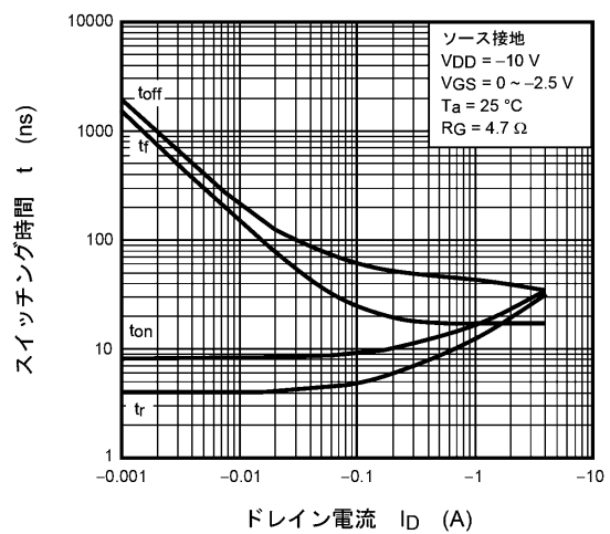
図 8.10 t - I_D
