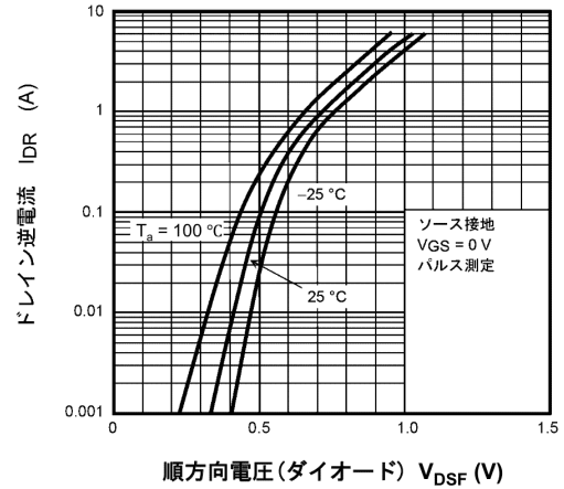
図 8.8 I_{DR} - V_{DSF}
