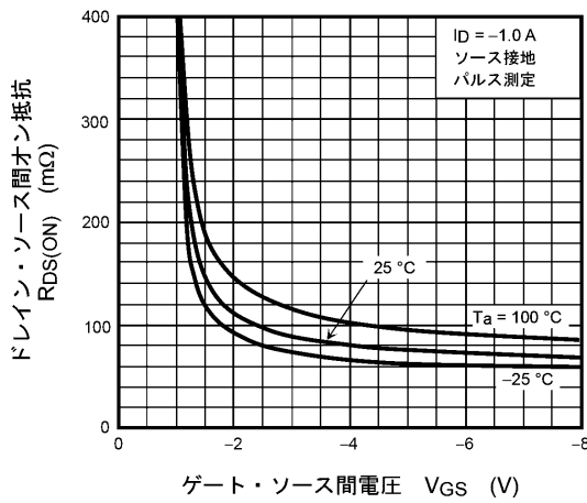
図 8.3 R_{DS(ON)} - V_{GS}
