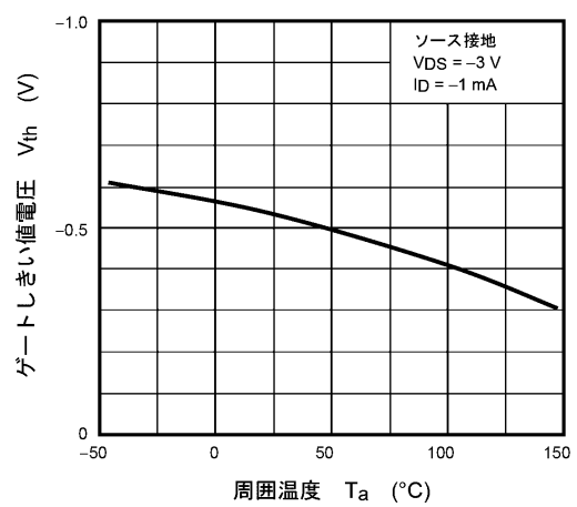
図 8.6 V_{th} - T_a
