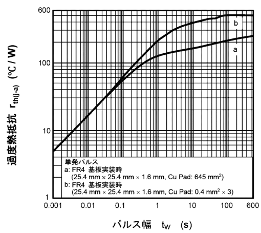
図 8.12 r_{th(j-a)} - t_w
