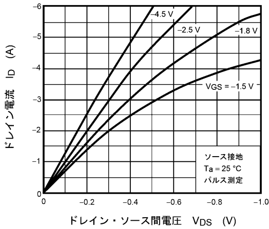
図 8.1 I_D - V_{DS}
