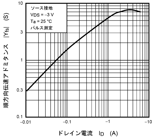
図 8.7 |Y_{fs}| - I_D
