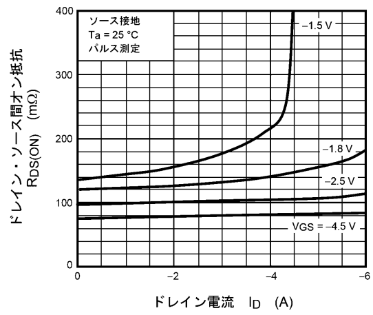
図 8.4 R_{DS(ON)} - I_D
