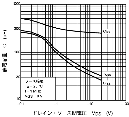
図 8.9 C - V_{DS}
