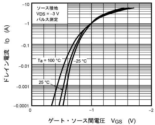
図 8.2 I_D - V_{GS}
