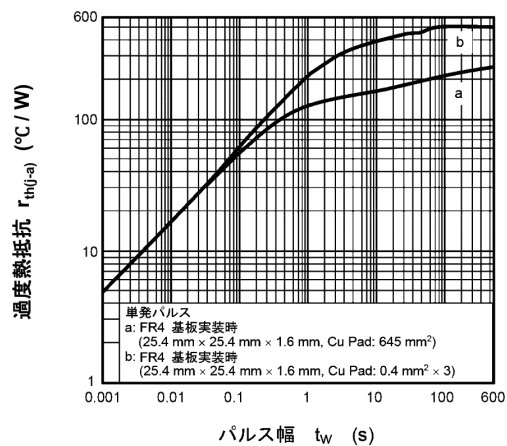
図 8.13 r_{th(j-a)} - t_w
