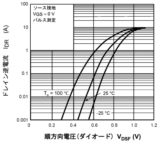
図 8.9 I_{DR} - V_{DSF}
