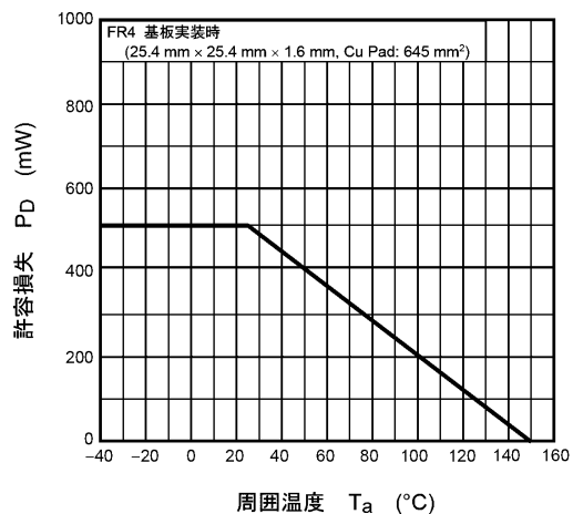
図 8.14 P_D - T_a
