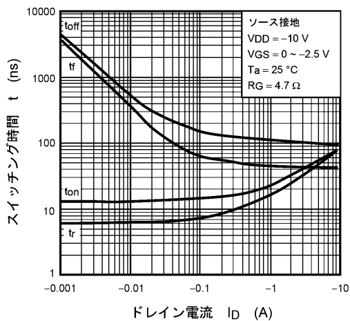
図 8.11 t - I_D
