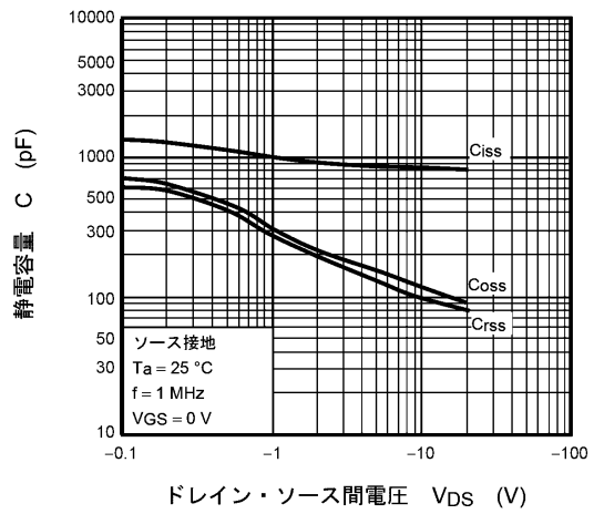
図 8.10 C - V_{DS}
