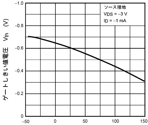
図 8.7 V_{th} - T_a
