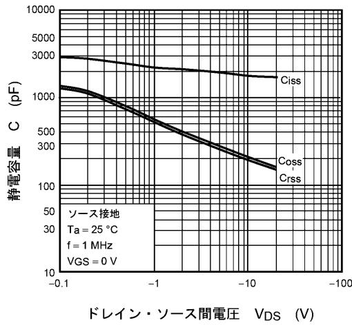
ドレイン・ソース間電圧 V_{DS} (V) 図 8.9 C - V_{DS}
