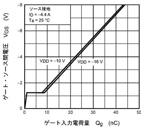
ゲート・ソース間電圧 V_{GS} (V) 図 8.11 ダイナミック入力特性
