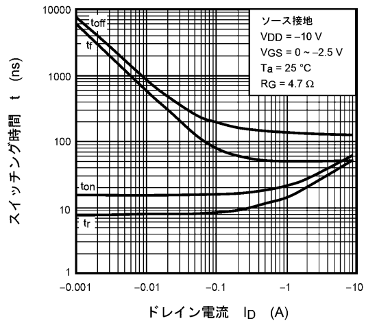
ドレイン電流 I_D (A) 図 8.10 t - I_D
