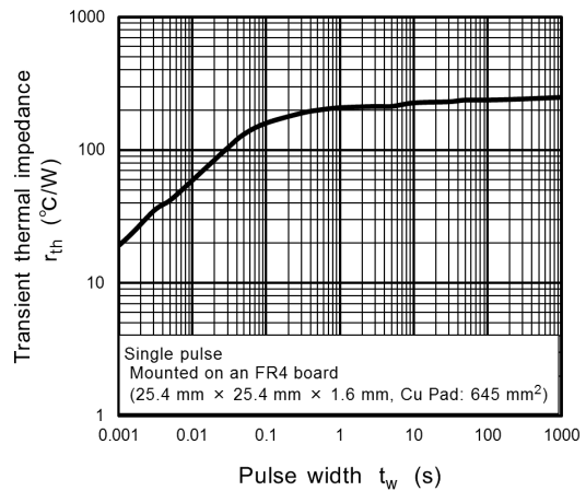
Fig. 8.10 r_{th} - t_w
