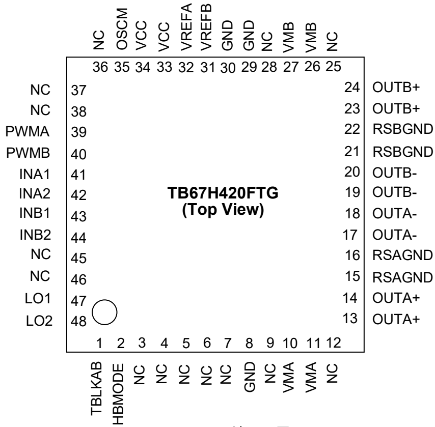
図 3.1 端子配置図
