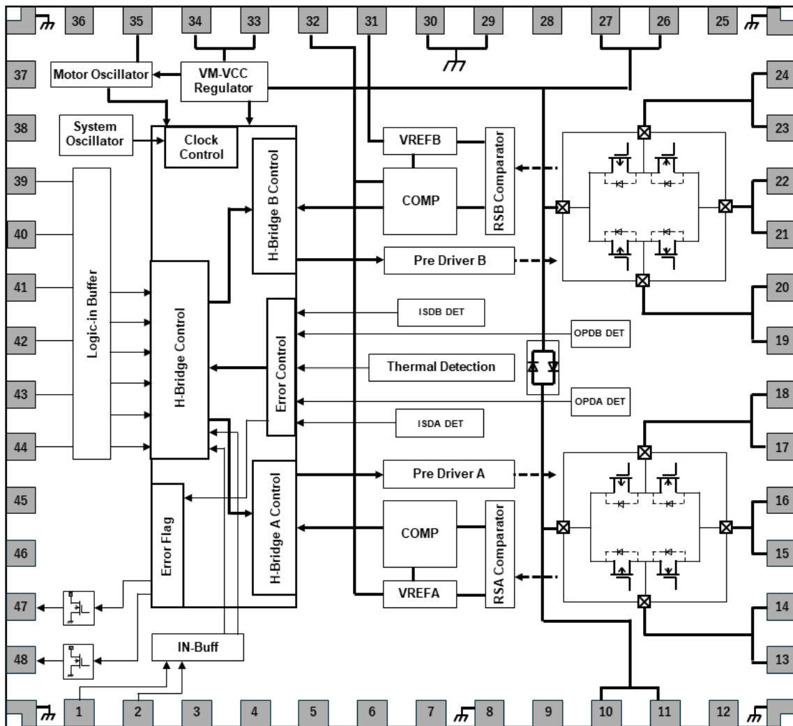
図 5.1 ブロック図
