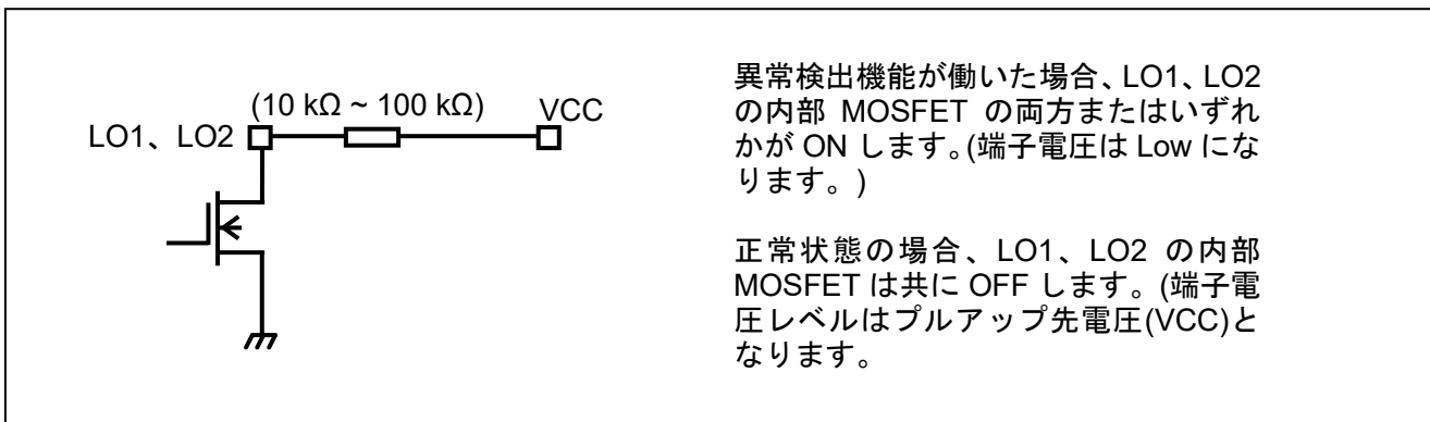
図 7.5 LO ファンクション等価回路
