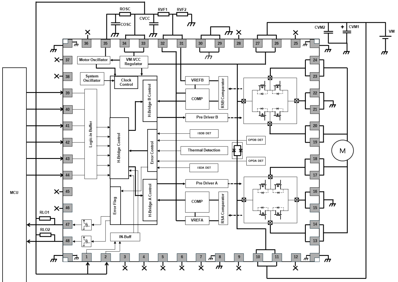
図 11.1 応用回路例
