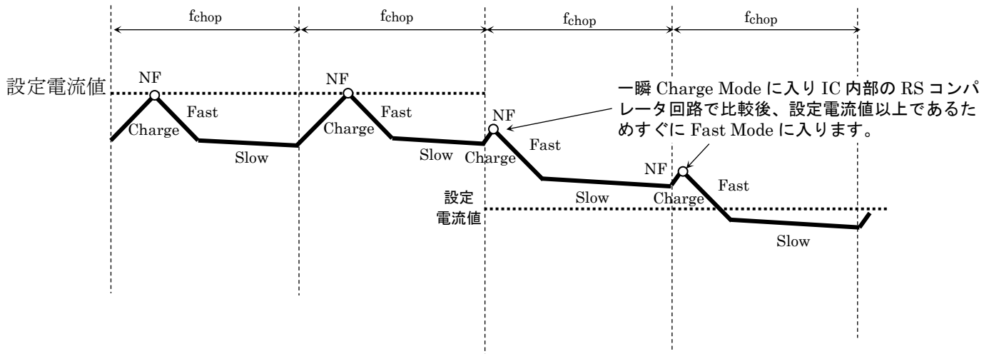
図 7.11 設定電流値が減少方向の場合
