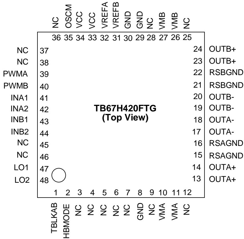
図 3.1 端子配置図
