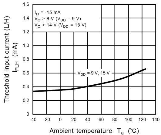
Fig. 12.2.2 I_{FLH} - T_a
