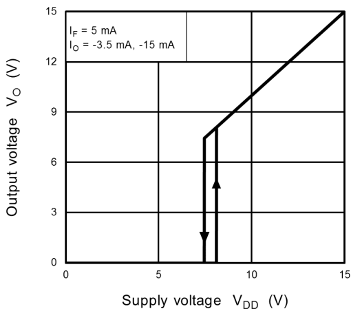
Fig. 12.2.11 V_O - V_{DD}
