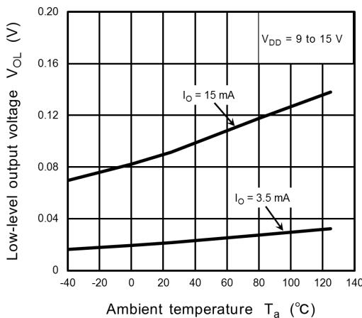
Fig. 12.2.5 V_{OL} - T_a
