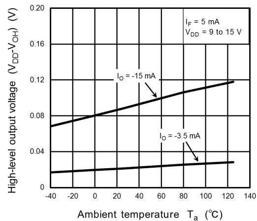
Fig. 12.2.6 (V_{DD} - V_{OH}) - T_a
