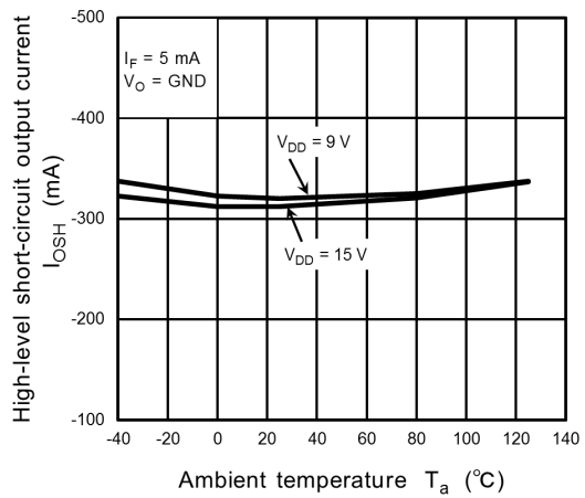
Fig. 12.2.10 I_{OH} - T_a
