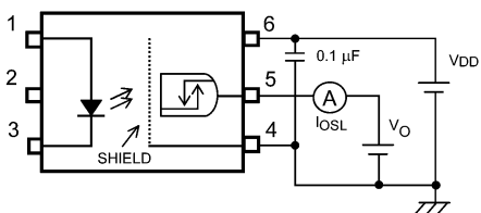
図 12.1.5 IOSL測定回路
