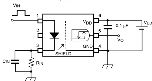
図 12.1.7 伝搬遅延時間測定回路, 波形
