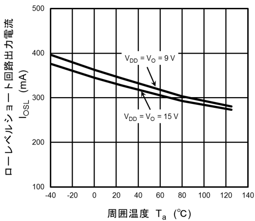
図 12.2.9 I_{OL} - T_a
