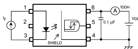
図 12.1.4 ICCH測定回路
