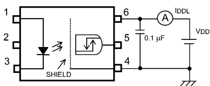
図 12.1.3 ICCL測定回路
