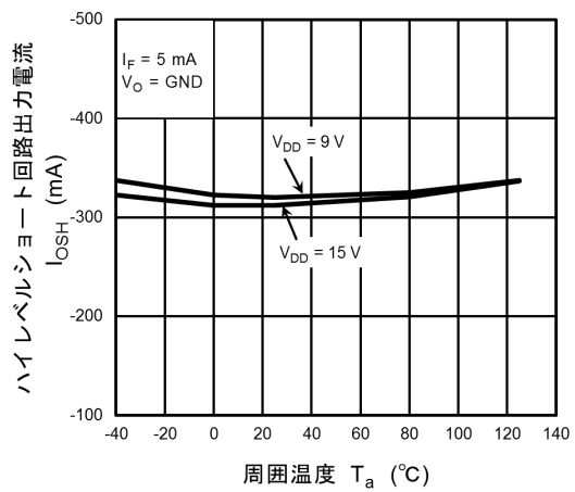
図 12.2.10 I_{OH} - T_a
