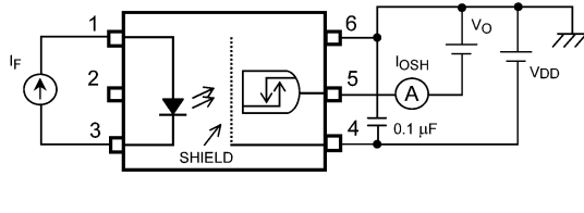
図 12.1.6 IOSH測定回路
