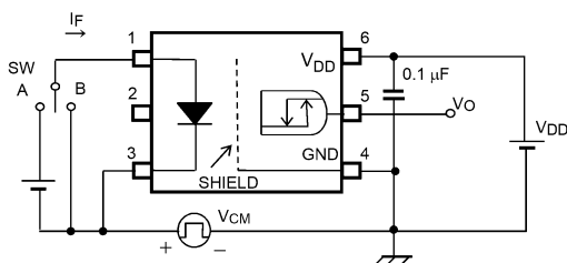
図 12.1.8 コモンモードノイズ除去電圧測定回路, 波形
