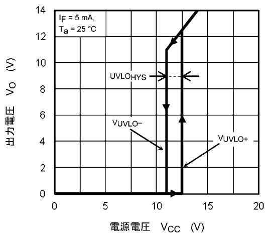
図 12.2.11 V_o(V_{UVLO}) - V_{CC}
