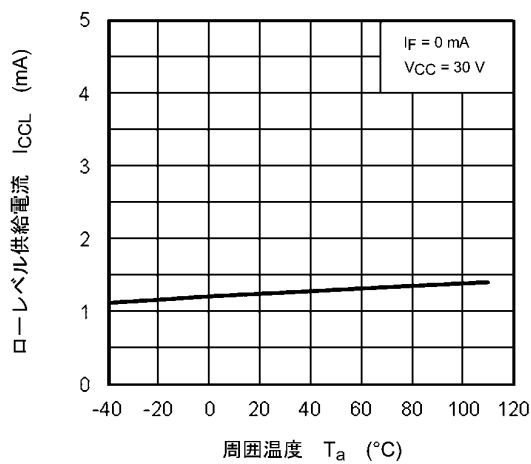
図 12.2.5 I_{CCL} - T_a
