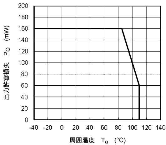
図 12.2.3 P_O - T_a
