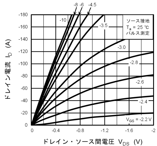
図 8.2 I_D - V_{DS}
