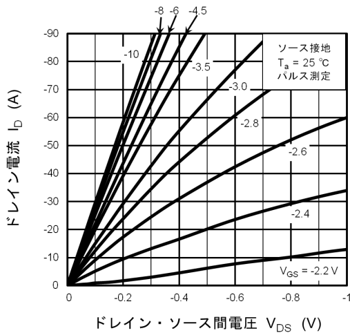
図 8.1 I_D - V_{DS}
