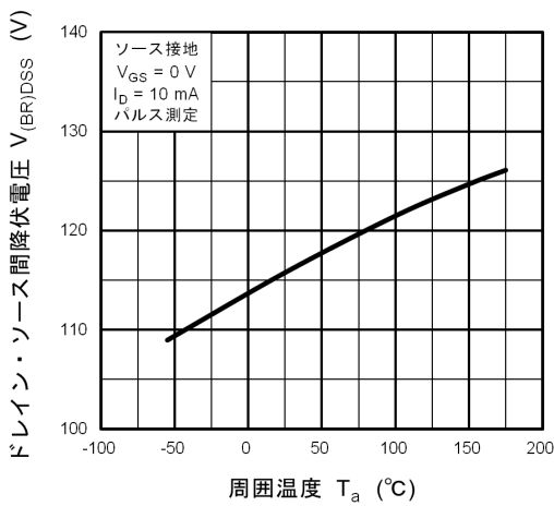
図 8.11 V_{(BR)DSS} - T_a
