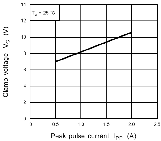
図 6.2.1 V_C - I_{PP}
