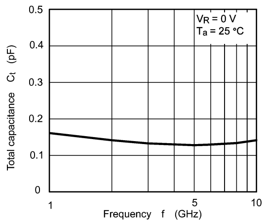
Fig. 9.4 C_t - f
