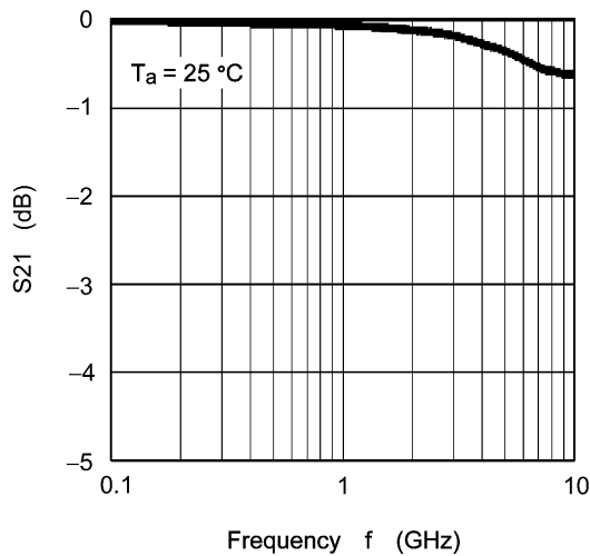
図 9.5 S_{21} - f
