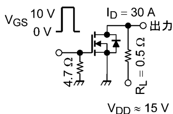
図 6.2.1 スwitchング時間の測定回路
