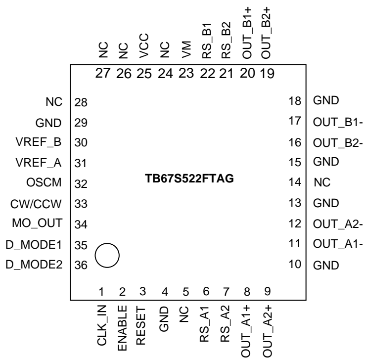
图 4.1 端子配置图
