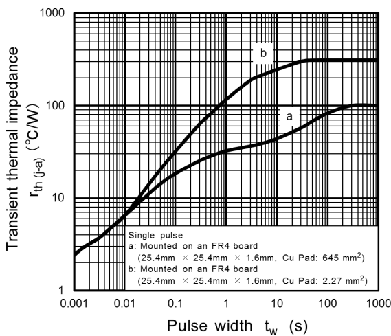
Fig. 9.11 r_{th} - t_w
