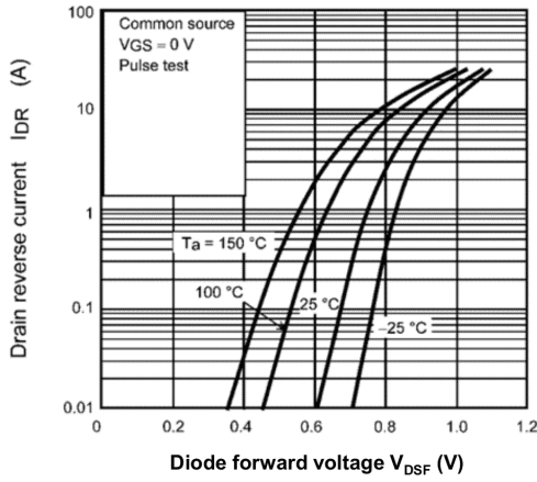
Fig. 9.7 I_{DR} - V_{DSF}
