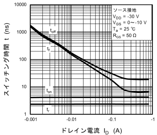
図 8.10 t - I_D
