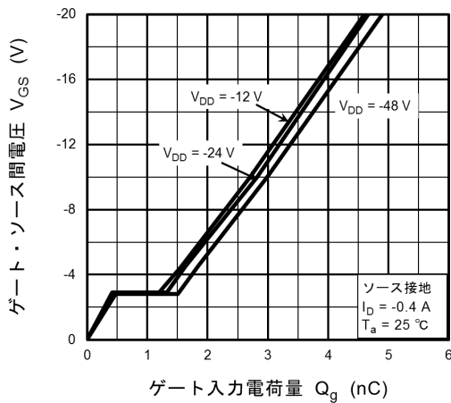
図 8.9 ダイナミック入力特性
