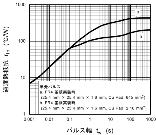
図 8.11 r_{th} - t_w
