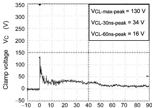
Pulse time t_p (ns) Fig. 6.1.3 +15 kV
