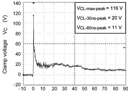
Pulse time t_p (ns) Fig. 6.1.1 +8 kV
