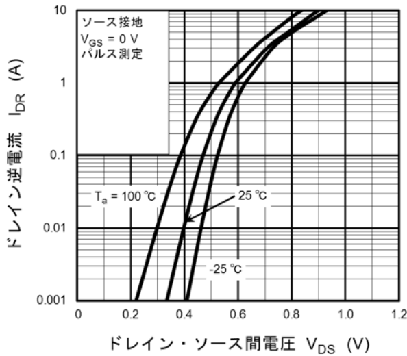
図 8.7 I_{DR} - V_{DS}
