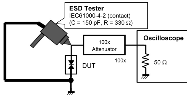
図 5.1.3 IEC61000-4-2 (Contact)
