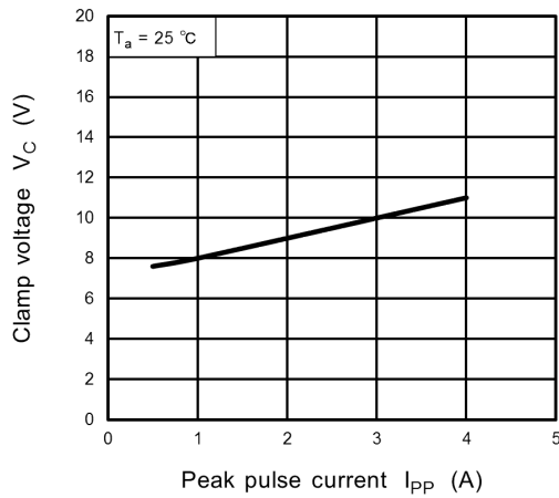
図 5.3.1 V_C - I_{PP}
