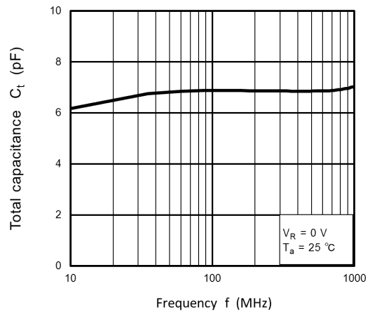
図 8.4 C_t - f
