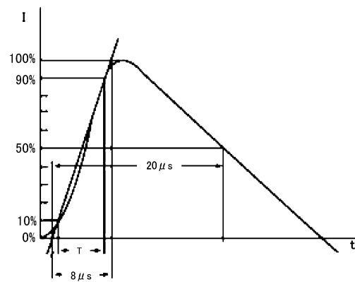
図 5.3.2 IEC61000-4-5準拠 8/20 \mu\text{s}
