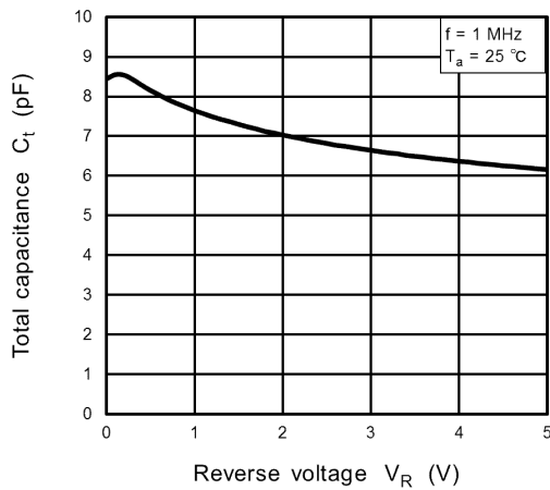
図 8.3 C_t - V_R
