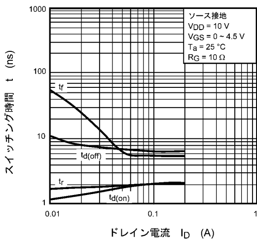
図 7.11 t - I_D
