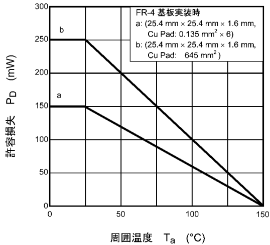
図 7.13 P_D - T_a
