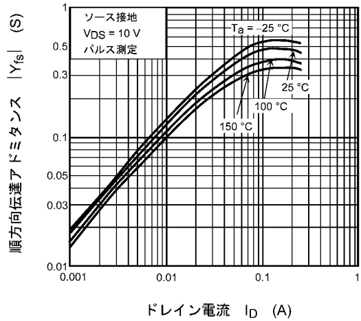
図 7.8 |Y_{fs}| - I_D
