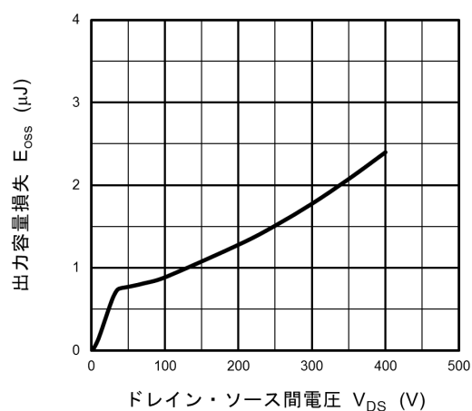
図 8.10 E_{OSS} - V_{DS}
