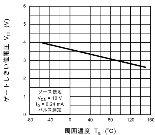
図 8.11 V_{th} - T_a
