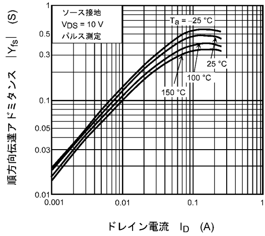
図 7.8 |Y_{fs}| - I_D
