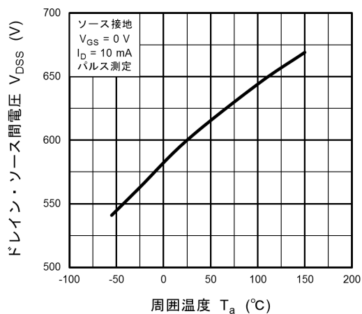
図 8.5 V_{DSS} - T_a
