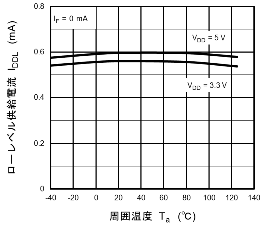
図 12.2.8 I_{DDL} - T_a
