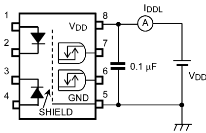
図 12.1.3 IDD_L測定回路
