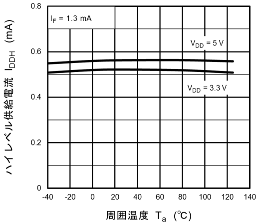
図 12.2.7 I_{DDH} - T_a
