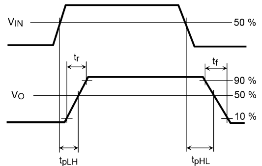
図 12.1.5 伝搬遅延時間測定回路, 波形
